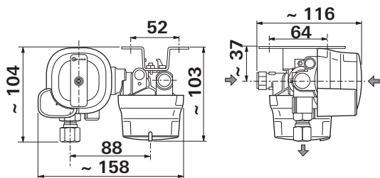
Slika 1a: Vertikalna naprava DuoControl
