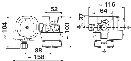
Obrázok 1a: DuoControl vertikálny
