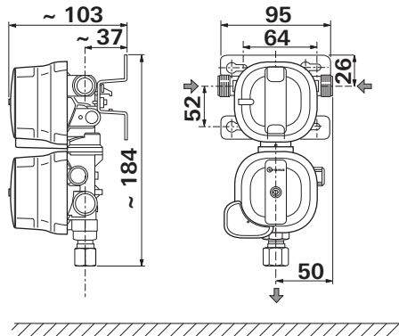
Obrázok 1a: DuoControl vertikálny
