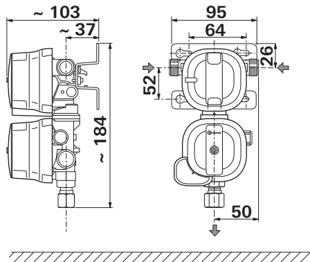
Imagem 1a: DuoControl vertical
