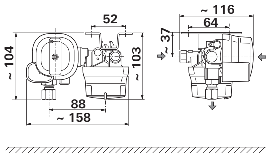
Imagem 1b: DuoControl horizontal Dimensões em mm. Representação não em escala. Fluxo de gás na direção da seta.
